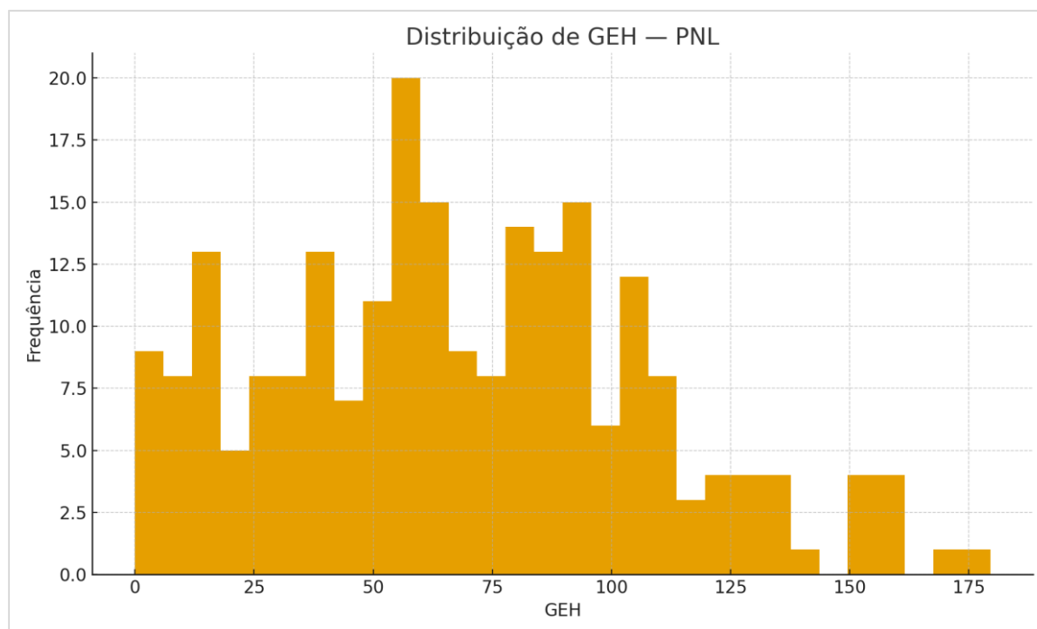
Figura F-4: Histograma de GEH (PNL 2050). Fonte: Consórcio Concremat-Transplan
