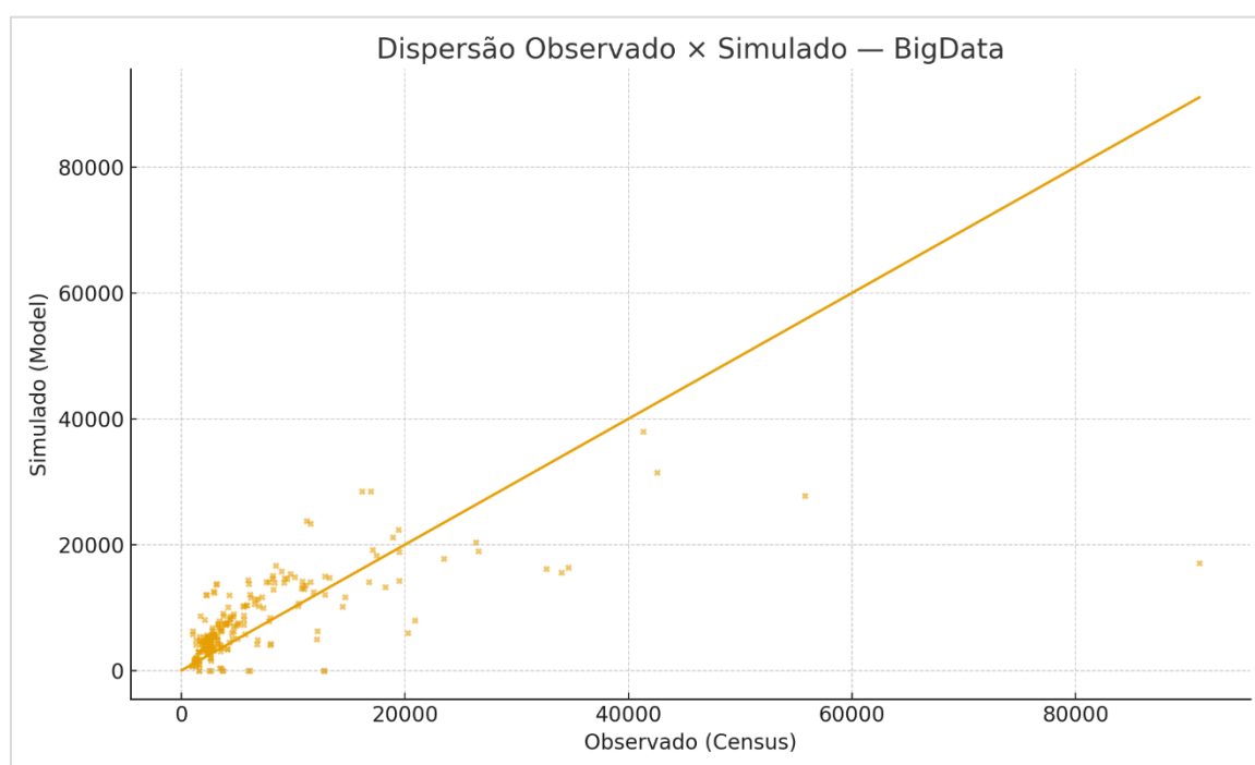
Figura F.1: Dispersão Observado x Simulado (Projeto Big Data). Fonte: Consórcio Concremat-Transplan
